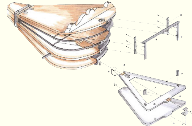
Planung einer Stützkonstruktion für einen Blasebalg von 1669
